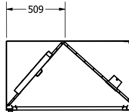
Sec a-a
